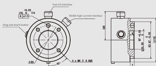
AUBO-i3 End Flange
