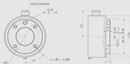
AUBO-i5 End Flange
