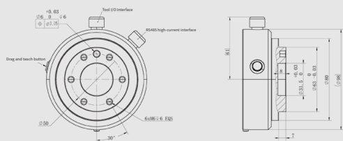
AUBO-iS20L End Flange
